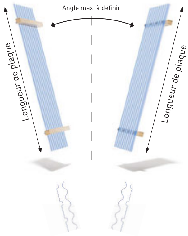
Pose inclinée
